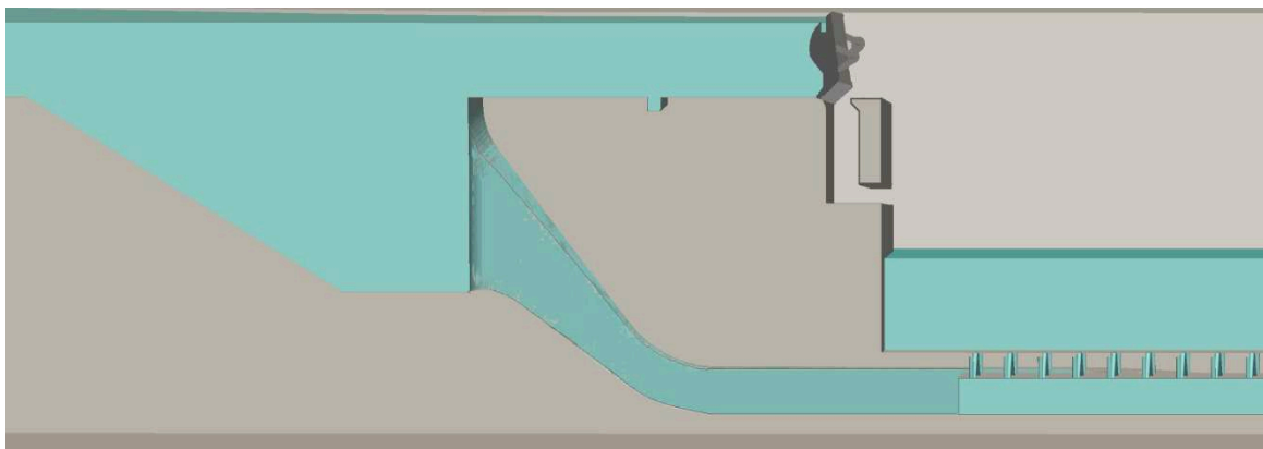
Bild 1 Bisher übliches Füllsystem für Fallhöhen > 10 m mit seitlichen Umlaufkanälen
