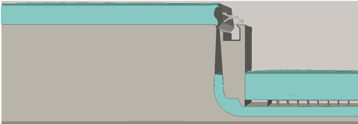
Bild 2 Neues vereinfachtes Füllsystem für Fallhöhen > 10 m mit horizontalem Fallschacht
