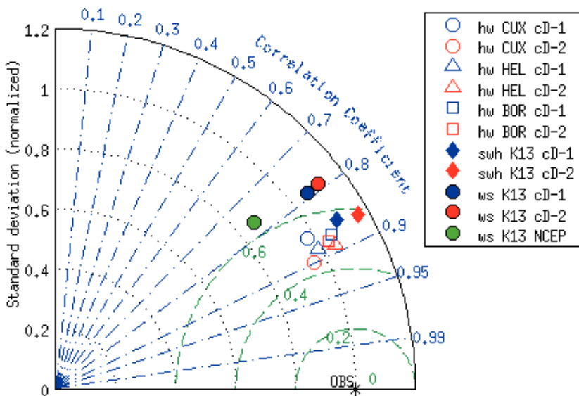
Abbildung 1: Taylor-Diagramm zum Vergleich der Ergebnisse aus coastDat-1 (blau) und coastDat-2 (rot) mit Beobachtungen. Ausgewertet wurden im Zeitraum von 2000 bis 2002 die Messgrößen Windgeschwindigkeit (gefüllte Kreise) und signifikante Wellenhöhe (gefüllte Rauten) an der Plattform K13 sowie Tidehochwasserstände in Cuxhaven (leere Kreise), Helgoland (leere Dreiecke) und Borkum (leere Quadrate). Für die Messgröße Windgeschwindigkeit ist zusätzlich ein Vergleich mit der antreibenden globalen NCEP-Reanalyse dargestellt (grün). Der schwarze Stern kennzeichnet die Position eines Datensatzes, der mit den Beobachtungen perfekt übereinstimmen würde.
