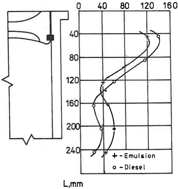
Bild 3 Verschleißergebnisse an den Zylinderbuchsen
