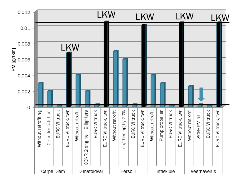
Bild 1: Partikelemissionen in g/tkm von fünf Binnenschiffen des MoVe IT!-Projekts verglichen mit jenen eines Sattelzuges (34 – 40 t) unter Berücksichtigung von Staubaufwirbelung und Abrieb des Straßenverkehrs ( PM_{10} ).
