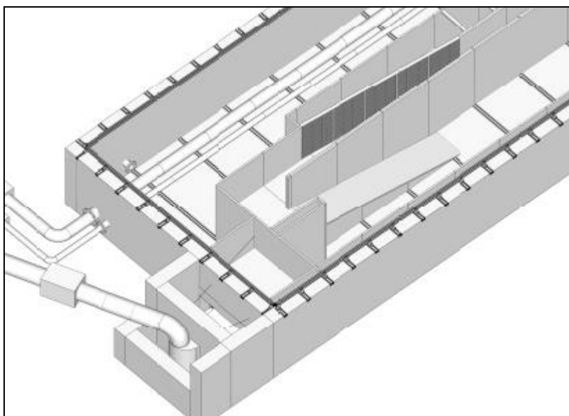
Abbildung 2: Konstruktionszeichnung des gegenständlichen Modells (Maßstab 1:5) zur Untersuchung des Einstiegsbereichs einer Fischaufstiegsanlage (Quelle: BAW)
