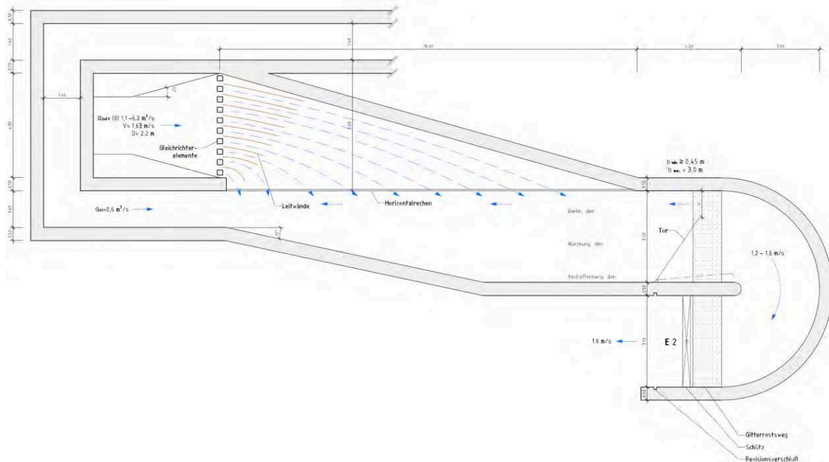
Abbildung 1: Skizze eines neuartigen Einstiegs in eine Fischeaufstiegsanlage (Quelle: ARGE)
