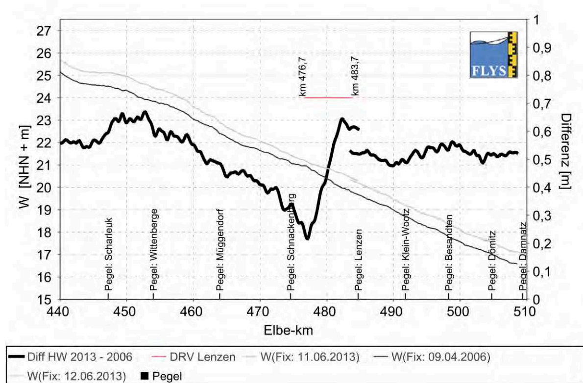
Abbildung 6: Gemessene Scheitelwasserspiegellagen an der unteren mittleren Elbe bei den Hochwassern Juni 2013 und April 2006 sowie die daraus resultierende Differenzlinie
