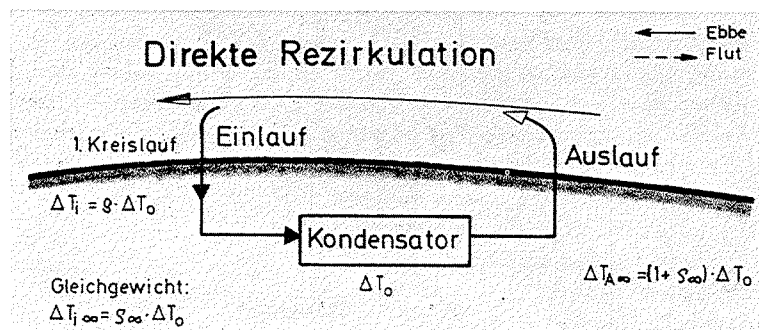
Abb. 2. Kühlwasserkreislauf eines Wärmekraftwerkes
