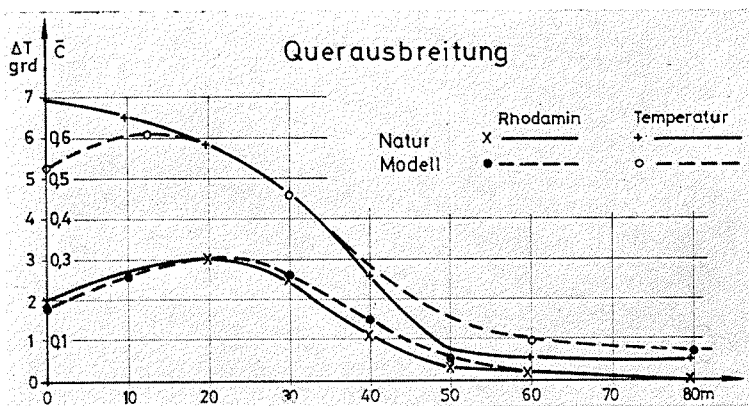
Abb. 7. Querverteilung 1\frac{1}{2} Stunden vor Tnw
