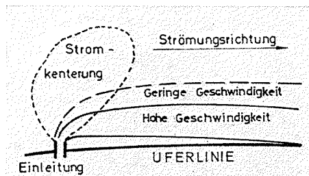
Abb. 6. Die Fahne bei verschiedenen Tidephasen
