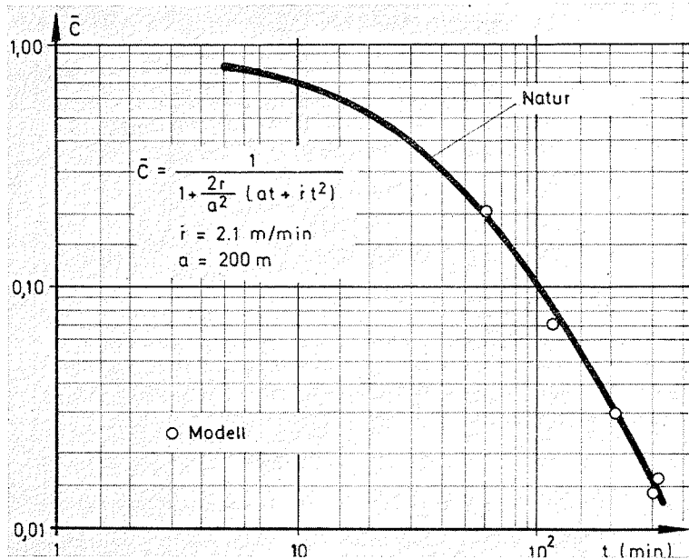
Abb. 8. Abnehmende Maximalkonzentration eines Farbflekes in Natur und Modell
