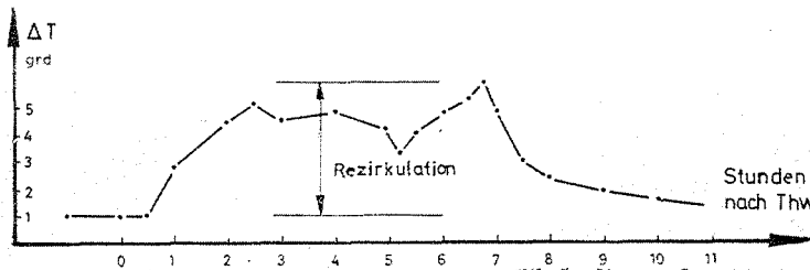
Abb. 3. Steigende Temperaturkurve während des Ebbstromes
