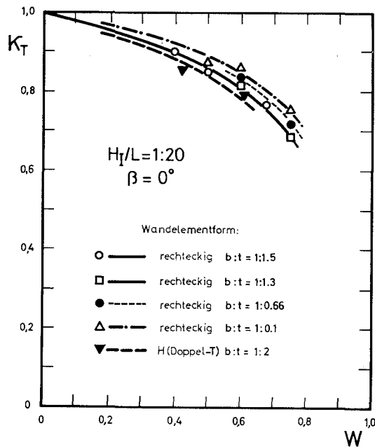
Abb. 8. Transmissionskoeffizient K_T als Funktion des Verbaunungsverhältnisses W
