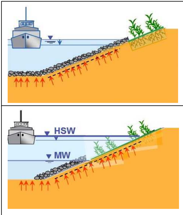
Bild 2: Anordnung pflanzliche Ufersicherungen an einem Kanal mit konstanten Wasserständen (oben), an einem Fluss mit schwankenden Wasserständen (unten)
