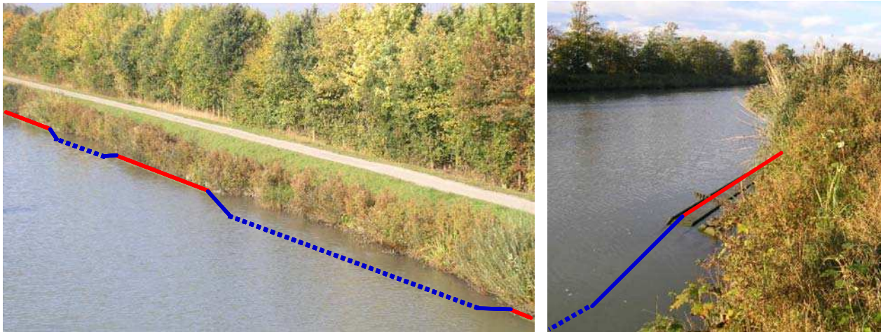
Bild 4.1: Versuchsstrecke MLK-km 189,5 bis 190,0, Nordufer Spundwand endet kurz über (rot) bzw. unter (blau) dem Wasserspiegel (BW o )
